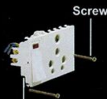
Switch & Socket Module
